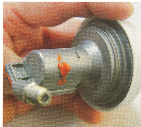
PLL-LNB Avenger (sans son capot)
