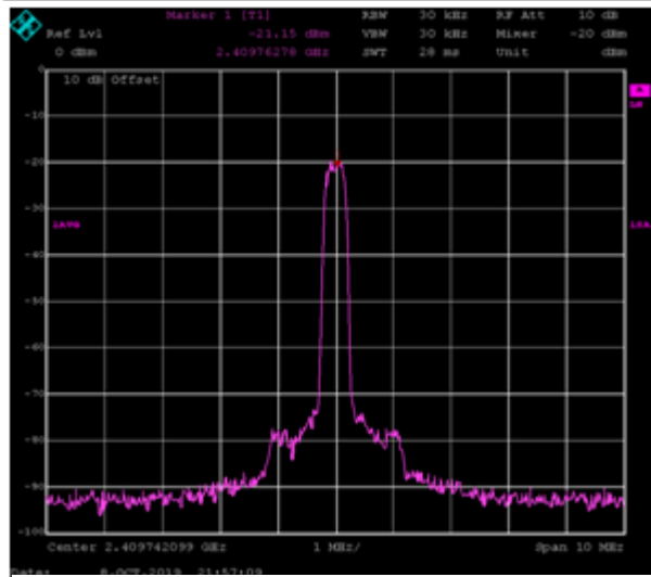
LNA4ALL + 10dB Pad on o/p
