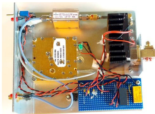
Fig 6 : Le module émetteur
