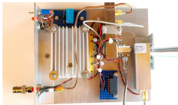
Fig 3 : Le module récepteur
