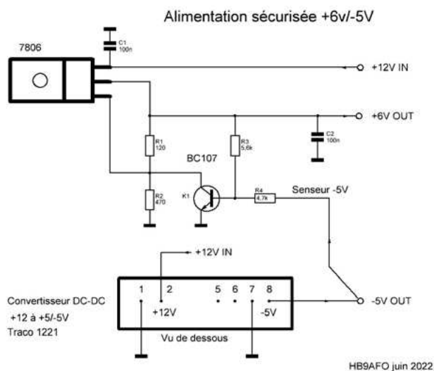
Fig 5 : Alimentation +6 et -5 V sécurisée
