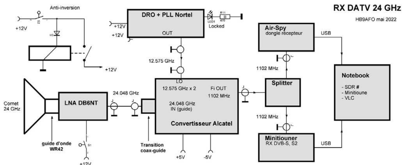
Fig 2 : Le schéma bloc de la réception
