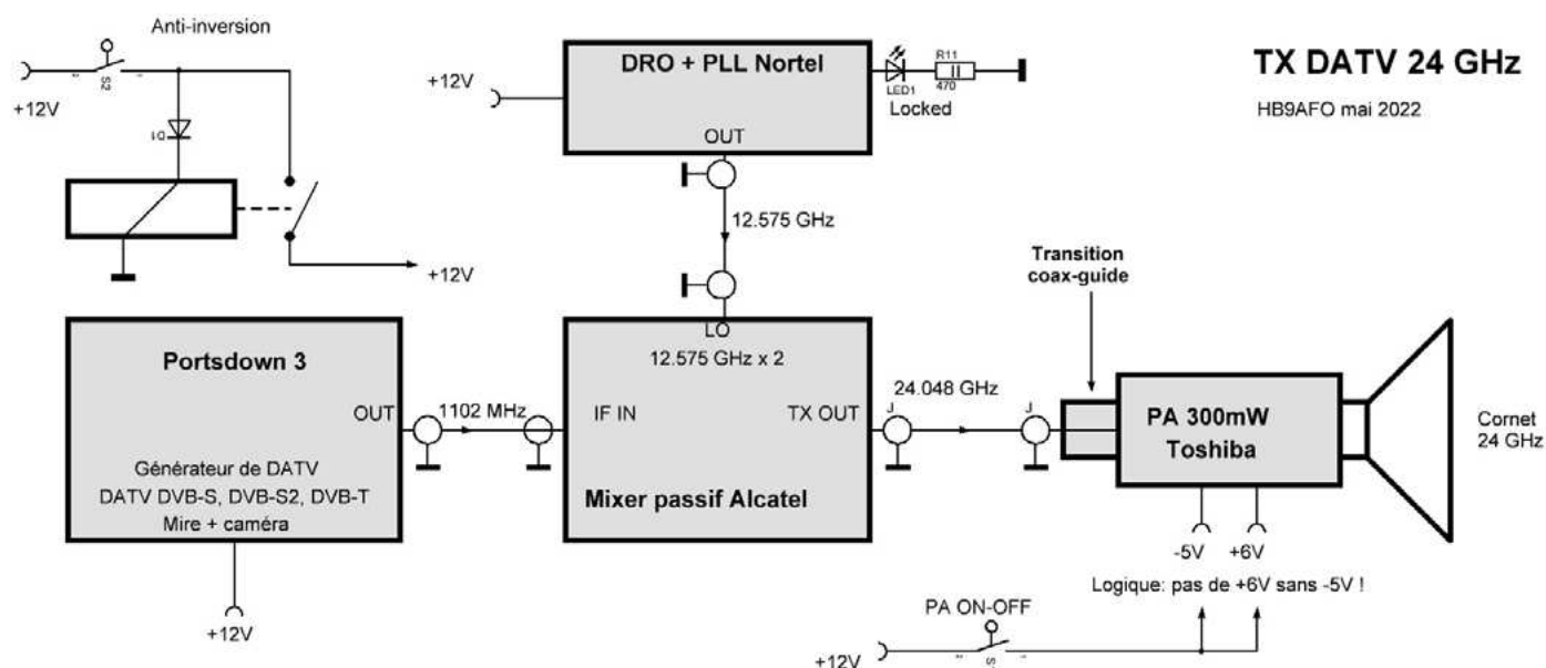
Fig 4 : Le schéma bloc de l'émission
